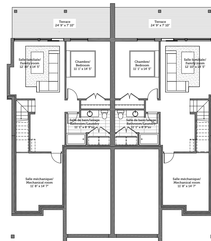
Niveau jardin/Garden level
